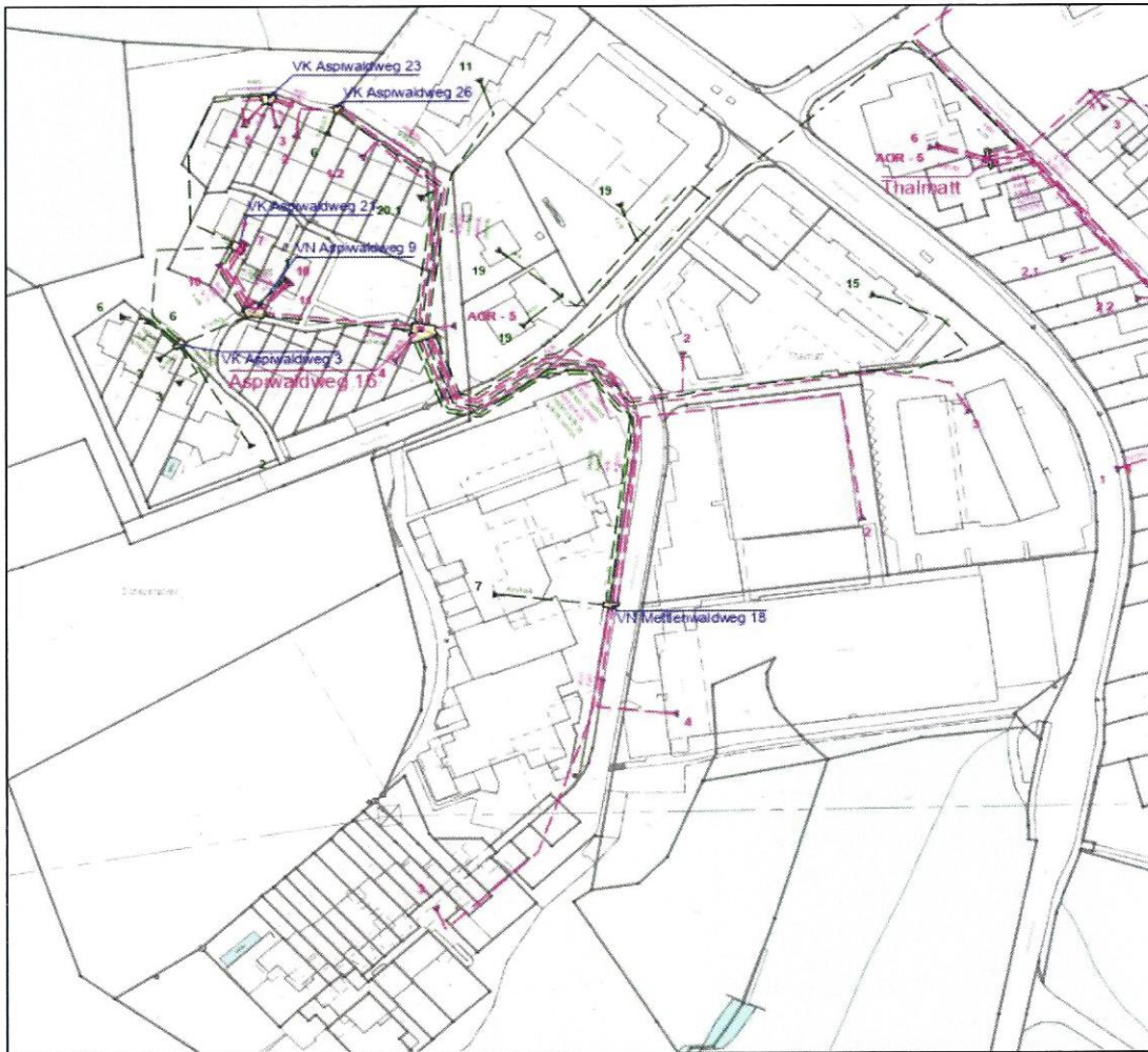
Ausschnitt vom Versorgungsgebiet Transformatorstation Aspiwaldweg 16
